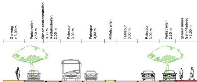
Musterquerschnitt Königsallee (1. BA) - Wohlfahrtstraße <> Wasserstraße
